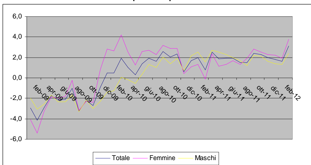
Graf.1 Variazione tendenziale dell'occupazione - periodo febbraio 2009-marzo 2012
