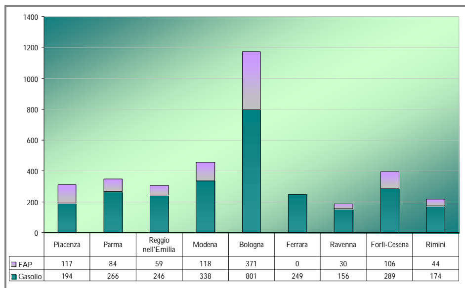
Figura 4 - Confronto Diesel e FAP nel parco circolante (Anno 2008)
