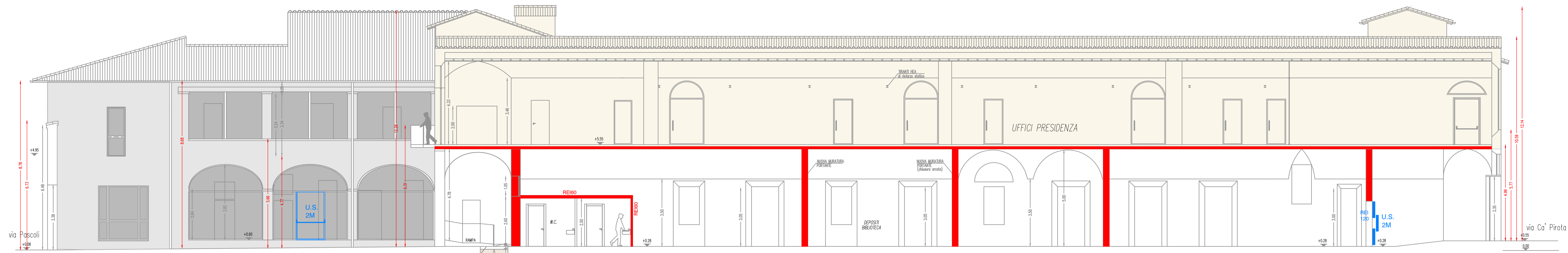
SEZIONE C-C Scala 1:100
