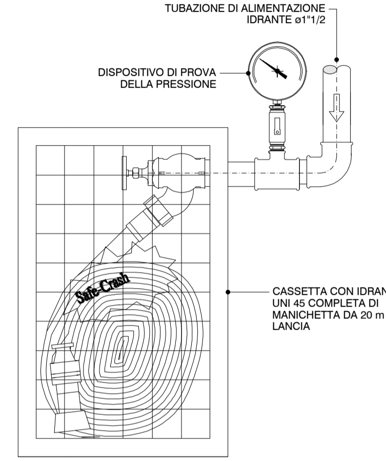
DETTAGLIO IDRANTE ANTINCENDIO UNI 45
